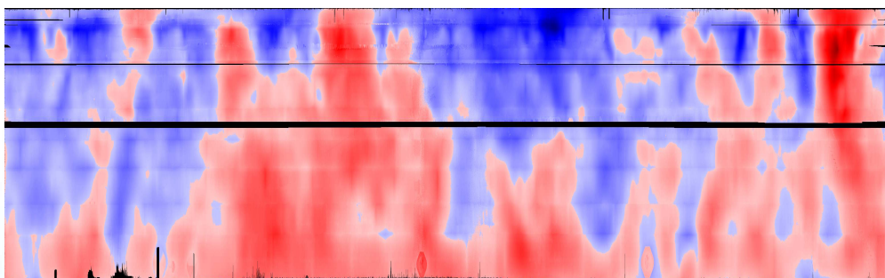
5 Dimnjak Urinj - oblak točaka i mapa ovalnosti
