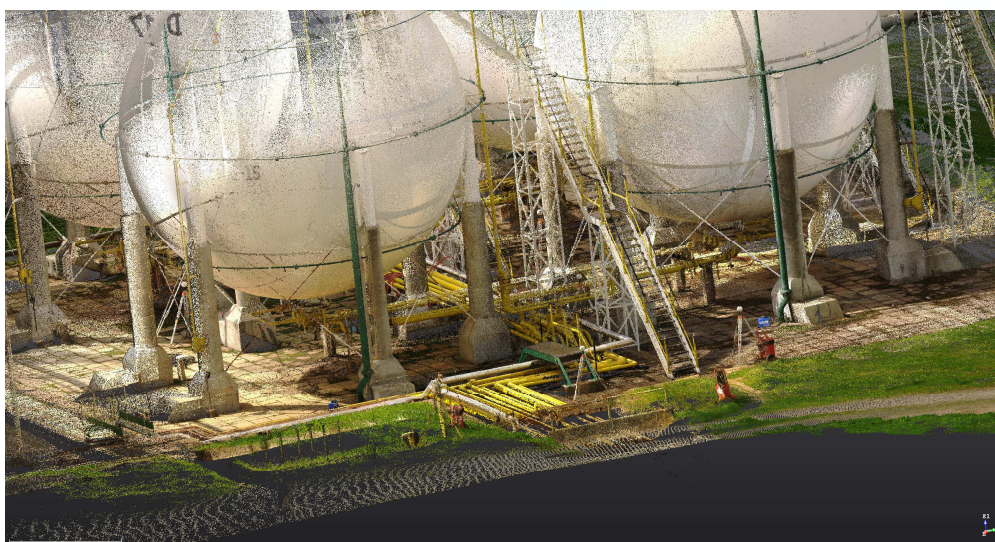
7 Spremnici ukapljenog plina - Point Cloud
