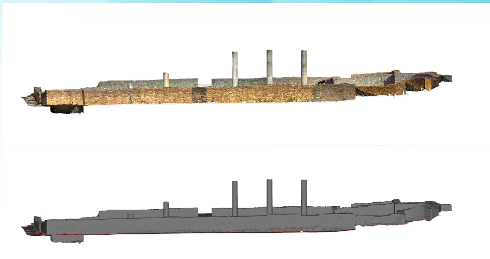
3 Projekcija oblaka i modela - Salona
